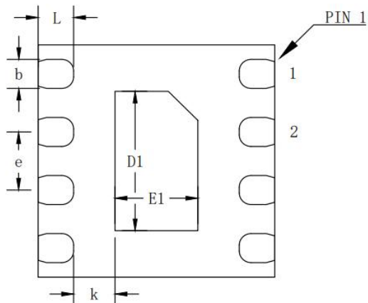
底视图
